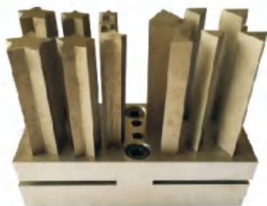
五角星/三角形冲压器 (15支) A star / Triangle (15 pcs)
